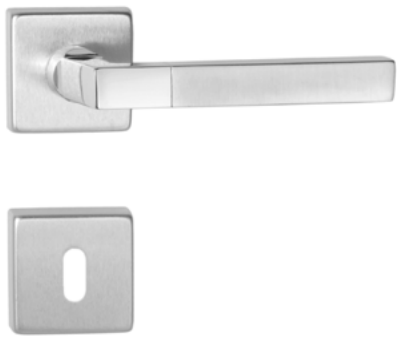
/// készleten ARIZONA F fényes króm és matt króm A zamak M A=125 mm D=50 mm
