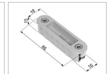
Alutop XT megfordítható zárólemez fém tokhoz Diszkrét, minimalista tervezésű műanyag zárólemez alumínium vagy más fém tokokhoz. Nem állítható, de 180°-ban megfordítva 1,5 mm-rel átpozicionálható a nyelvfogadó nyílása. Választható színek: szürke, matt fehér és matt fekete. Megrendelésre.
