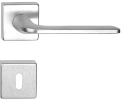
/// készleten OREGON négyzetrozettás, matt króm F matt króm A zamak M A=125 mm D=50x50 mm
